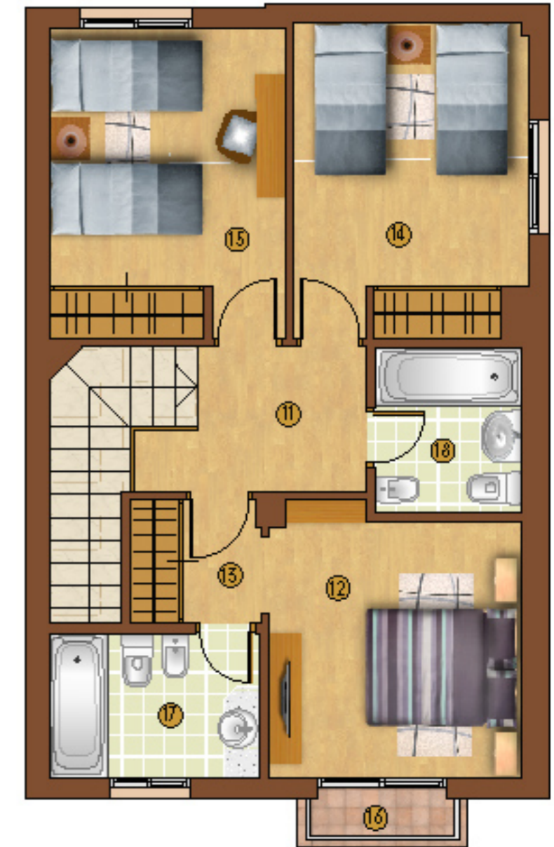
PLANTA ALTA
