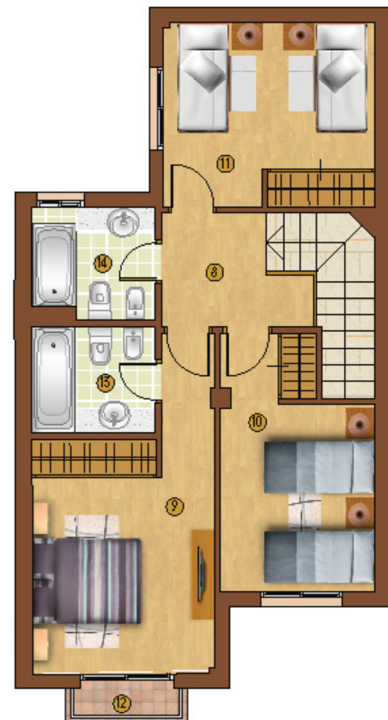
PLANTA ALTA
